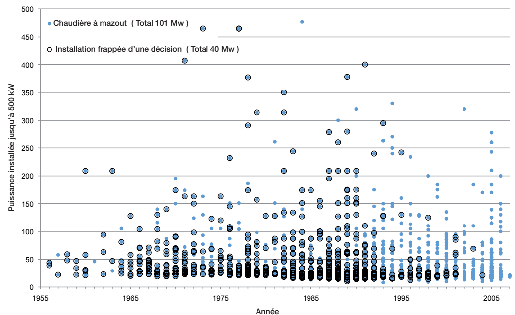
Illustration 6 : Puissance installée des installations de combustion par année de construction, installations frappées d'une décision d'assainissement comprises
