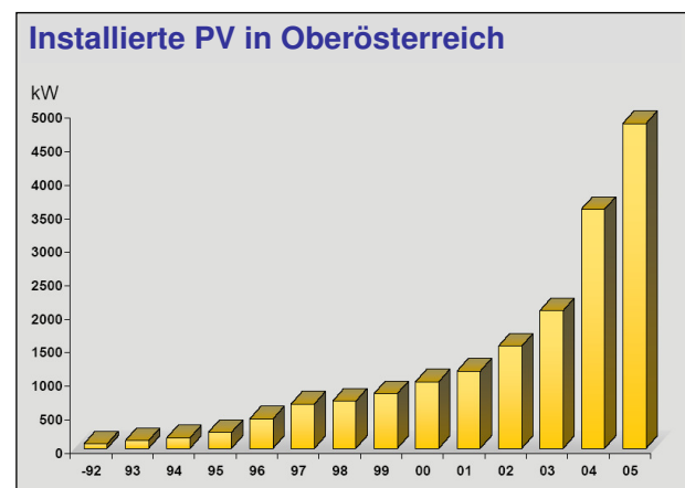
Abbildung 21: Entwicklung der Photovoltaikanlagen mit Netzeinspeisung in Oberösterreich
